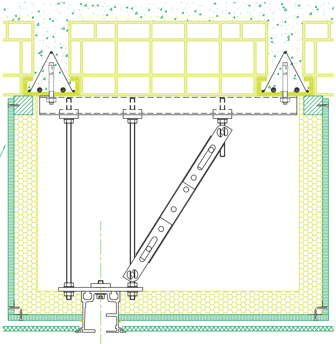
soluzione con controsoffitto solution with false ceiling
