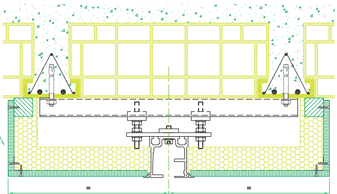
soluzione senza controsoffitto solution without false ceiling
