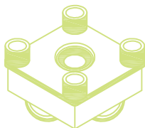
Tipo a CROCE per moduli bicarrello CROSS-shaped trolleys for bi-track modules
