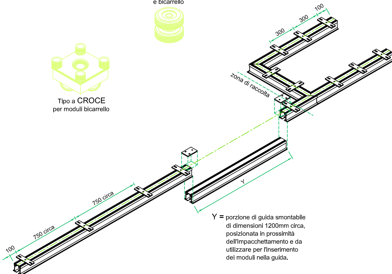
Tipo ASSIALE per moduli monocarrello e bicarrello
