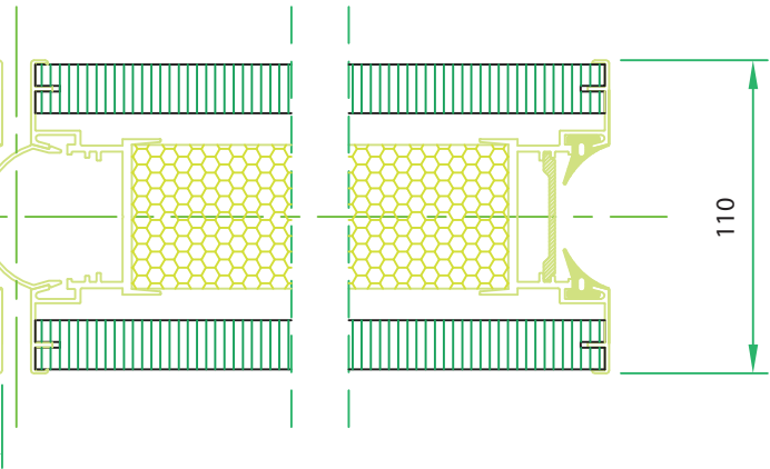
particolare modulo S con profili in vista su montante di partenza MP S module detail with visible profiles on the initial jamb MP
