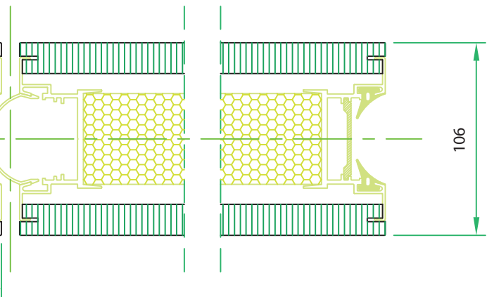
particolare modulo S con profili nascosti su montante di partenza MP S module detail with hidden profiles on the initial jamb MP
