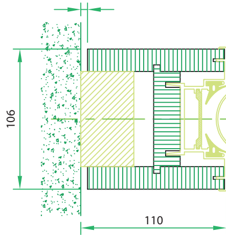
scuretto per recupero fuori piombo vertical alignment element
