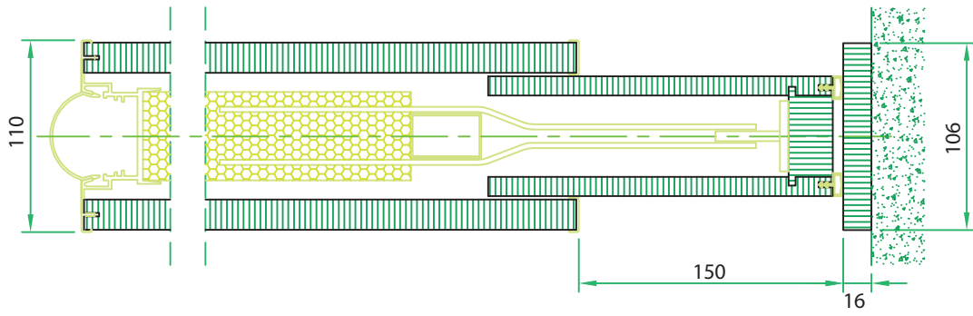
particolare modulo TC bicarrello con profili in vista su montante di arrivo MA TC bi-track module detail with visible profiles on the final jamb MA
