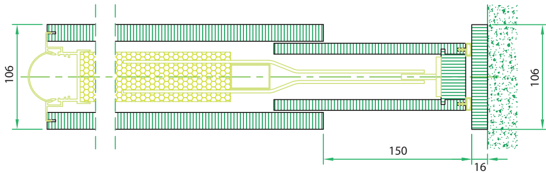
particolare modulo TC bicarrello con profili nascosti su montante di arrivo MA TC bi-track module detail with hidden profiles on the final jamb MA
