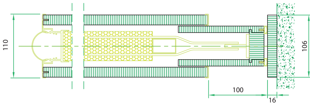
particolare modulo TC monocarrello con profili nascosti su montante di arrivo MA TC mono-track module detail with hidden profiles on the final jamb MA
