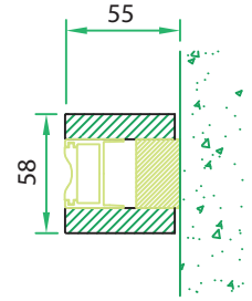
montante di partenza - arrivo initial / final jamb
