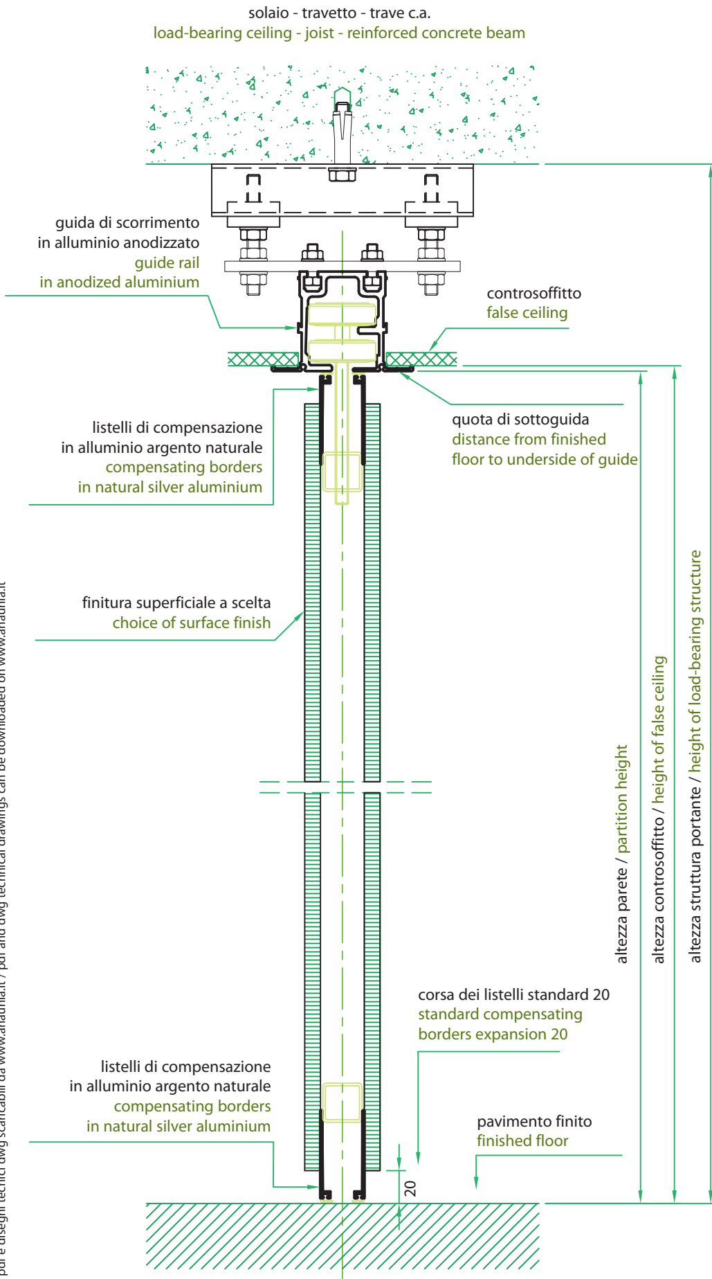
montante di partenza - arrivo initial / final jamb
