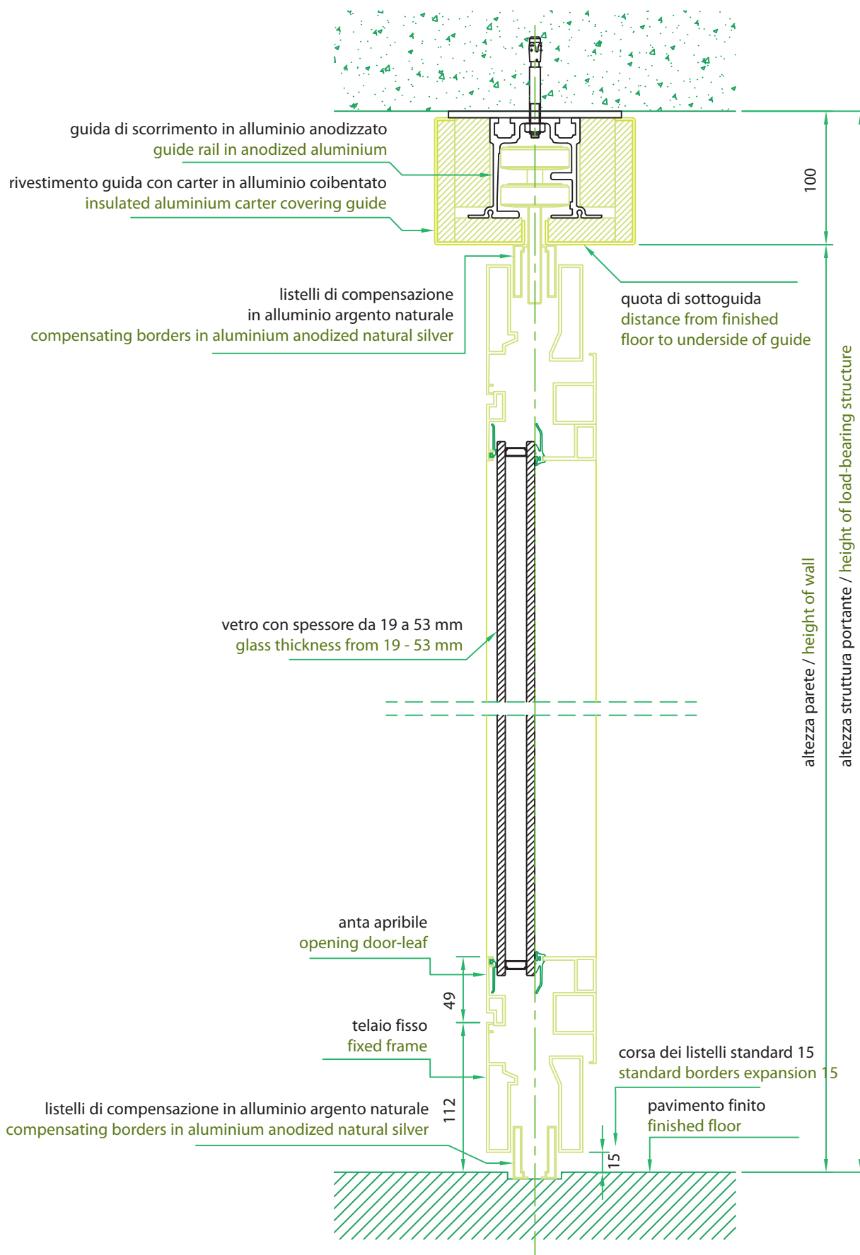
sezione su modulo porta-finestra solaio - travetto - trave c.a. section of glass door/window module - joist - reinforced concrete beam
